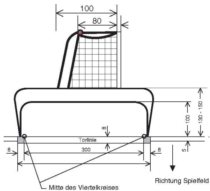
Abbildung 2b: Das Tor - Seitenansicht
